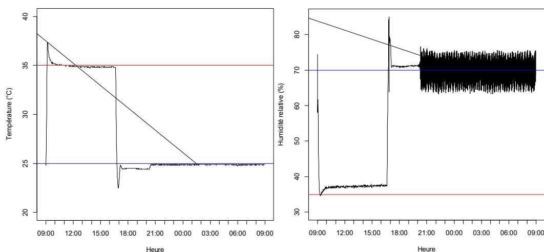
Figure 2 : Profil de la température (gauche) et de l'humidité relative (droite) dans l'enceinte climatique. Les droites rouge et bleue indiquent les consignes jour et nuit, respectivement.
